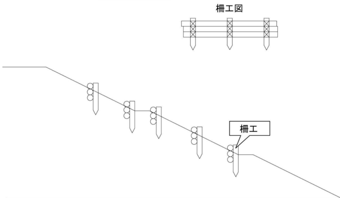
柵工施工図
