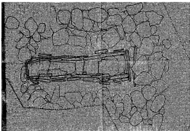
石ノ塔古墳実測図（群大史学研究室作図）
