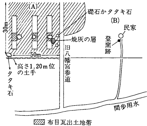
天代窯跡要図
